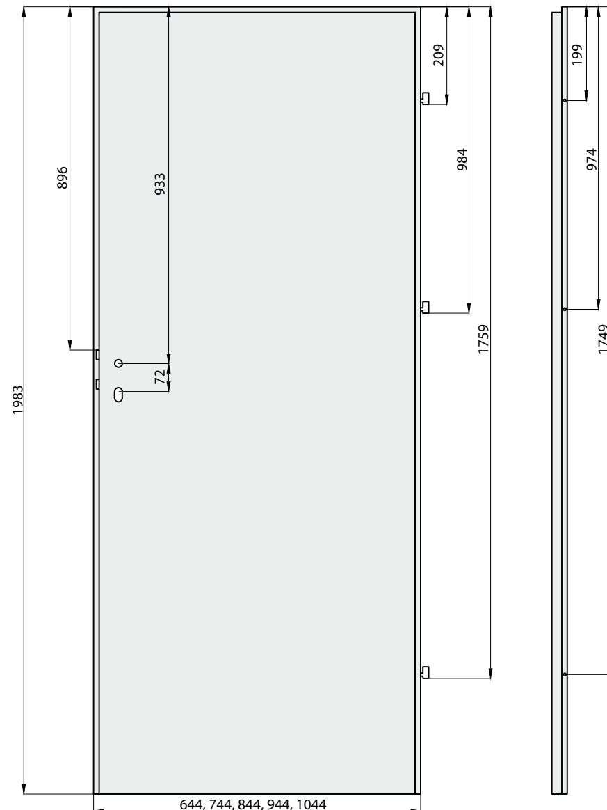
Nákras 1
